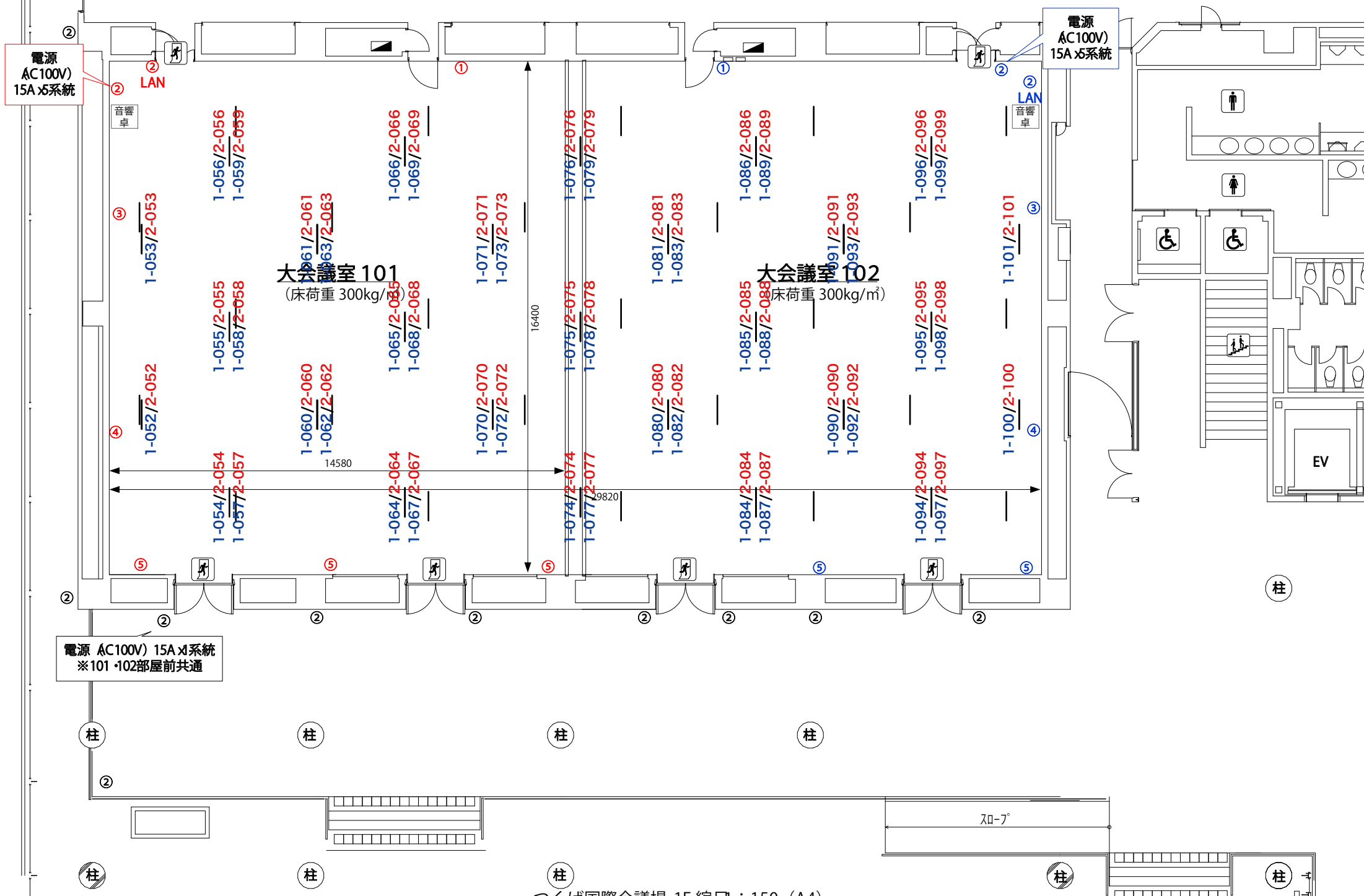
つくば国際会議場 1F 縮尺：150 (A4)
