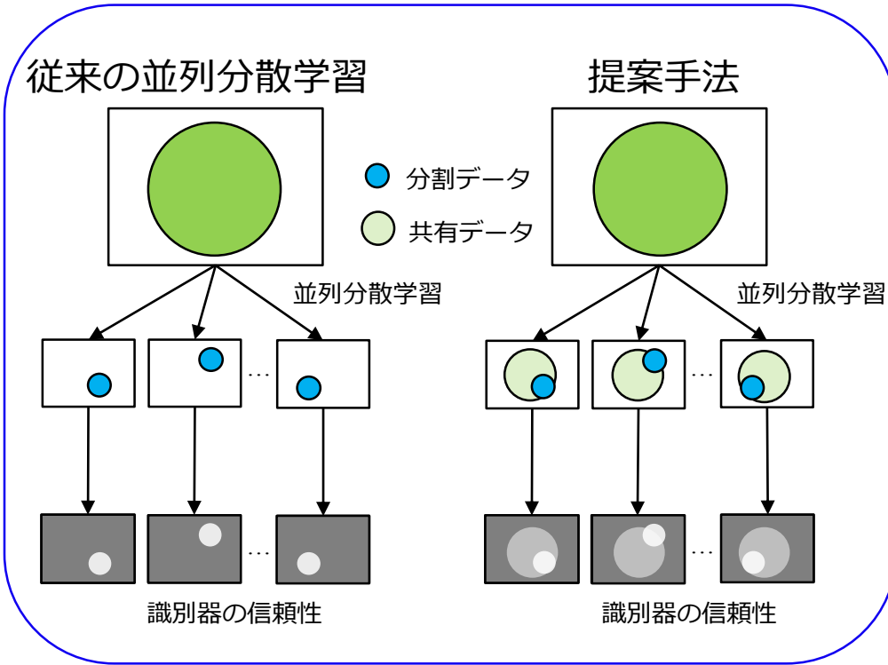
共有データによる過学習の抑制
