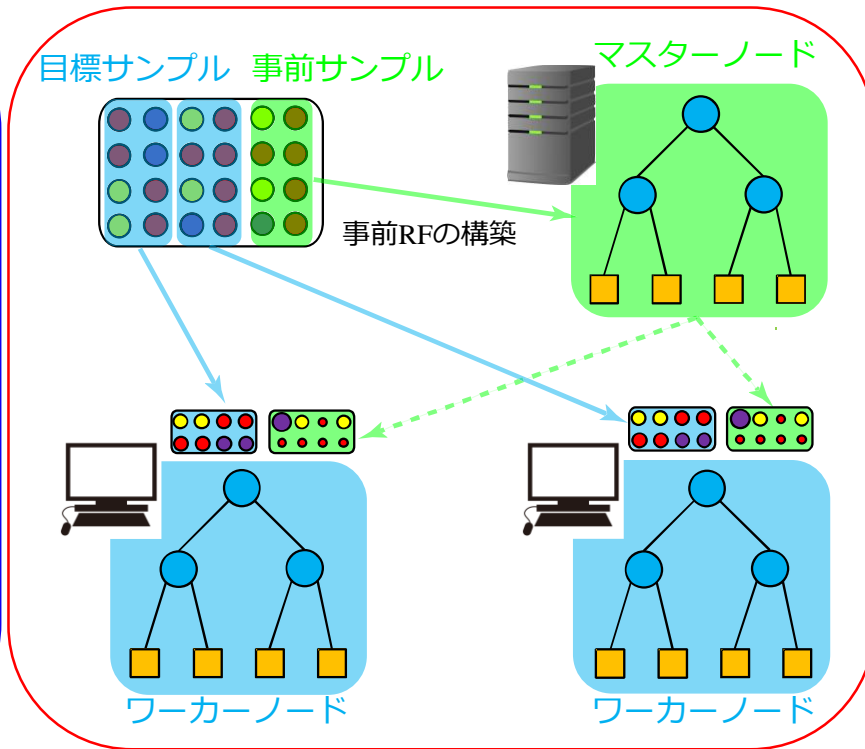
転移学習による共有データの学習の効率化
