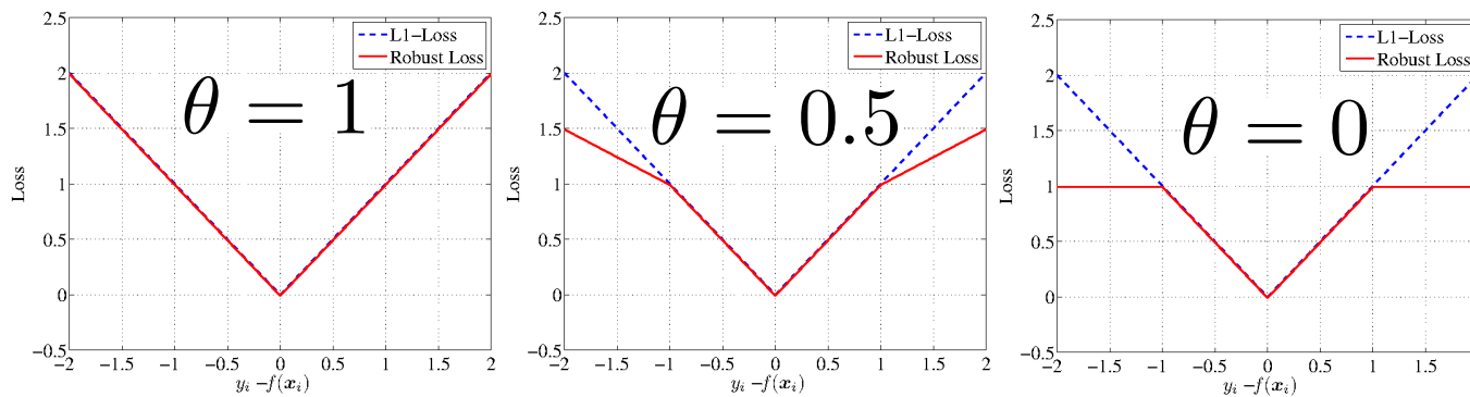
ロバストSVMの損失関数
